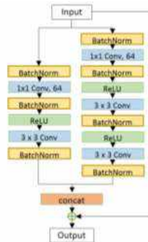
Hình 3. Kiến trúc khối residual cải tiến
