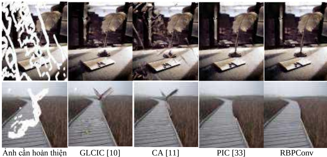
Hình 5. So sánh kết quả của RBPconv với các phương pháp trước đó
