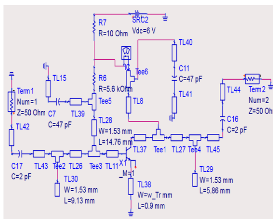
Hình 5. Mạch khuếch đại
