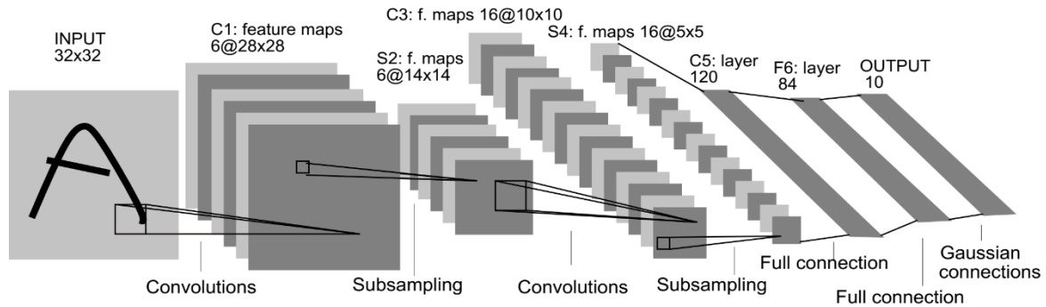
Hình 2. Kiến trúc mạng nơ-ron tích chập LeNet [7]
