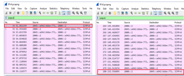
Hình 10. Bắt gói tin ICMPv6 của IPv6
