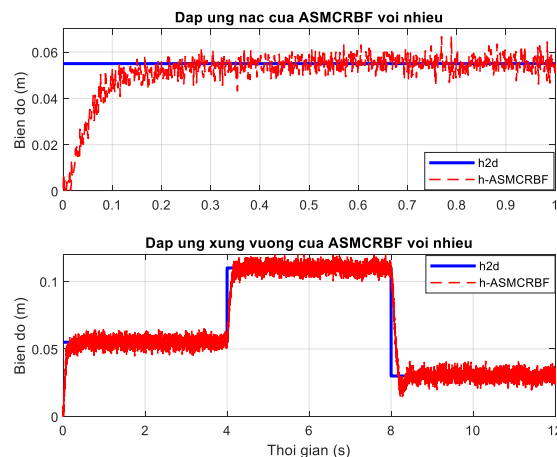
Hình 10. Đáp ứng với hàm nấc và xung vuông của bộ điều khiển ASMCRBF trong trường hợp nhiễu trắng tác động ở ngõ ra
