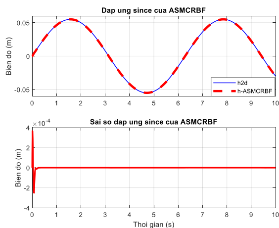
Hình 5. Đáp ứng since và sai số của bộ điều khiển ASMCRBF
