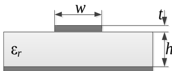
Hình 1. Cấu trúc đường truyền mạch dài
