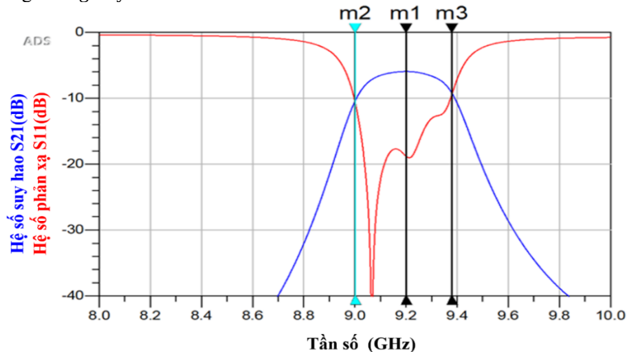
Hình 7. Hệ số phản xạ S_{11} và hệ số suy hao S_{21} của bộ lọc
