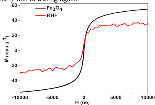
Hình 5. Đường cong từ trễ của vật liệu \text{Fe}_3\text{O}_4 và RHF
