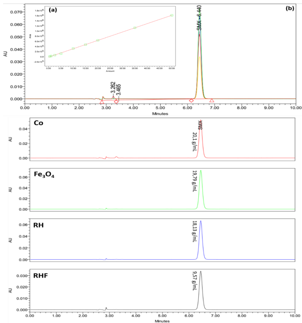
Hình 6. Đường chuẩn của SMX (a), chồng phổ HPLC của các vật liệu (b) và phổ HPLC của SMX sau khi hấp phụ bằng \text{Fe}_3\text{O}_4 , RH và RHF
