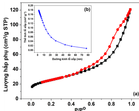
Hình 4. (a) Đường đẳng nhiệt hấp phụ - giải hấp phụ \text{N}_2 và (b) sự phân bố kích thước các lỗ xốp của vật liệu RHF
