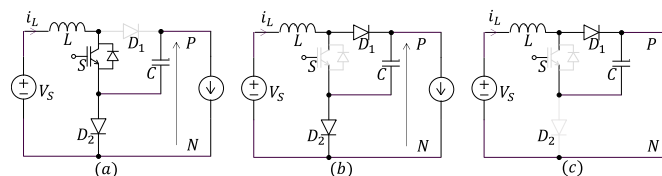
Hình 2. Chế độ vận hành của 3P2LqSBI (a) SB, (b) NSC and (c) ST
