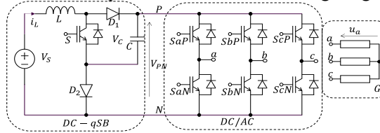
Hình 1. Sơ đồ nguyên lý nghịch lưu QSBI
