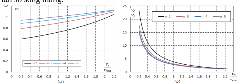
Hình 4. Đặc tính giảm điện áp stress và đặc tính tăng chỉ số điều chế m
