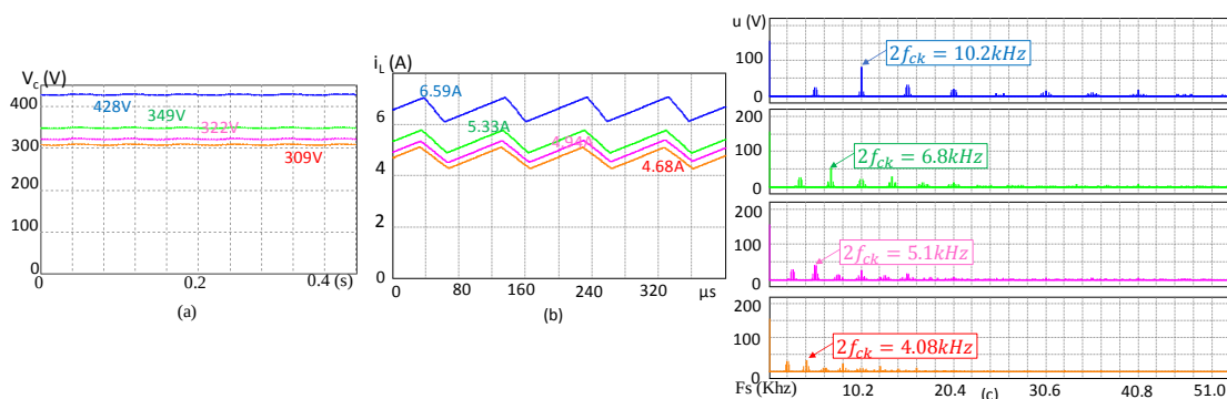
Hình 6. Kết quả mô phỏng với V_S=110V , v_{rms}=110V_{rms} các kỹ thuật nhiều sóng mang, nét vẽ xanh dương, xanh lá, tím và đỏ là tương ứng với kỹ thuật 2, 3, 4 và 5 sóng mang; (a) điện áp trên tụ DC link, (b) dòng điện ngõ vào là i_L và (c) phổ tần điện áp pha tải
