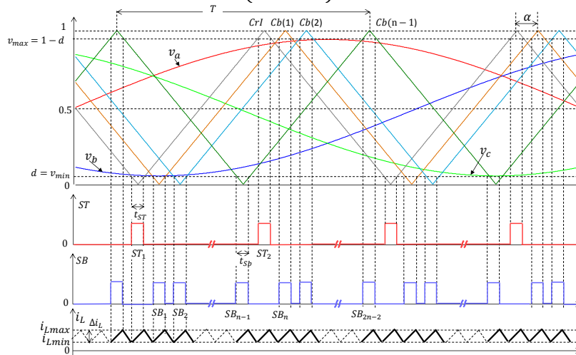
Hình 3. Nguyên lý điều khiển qSBI nhiều sóng mang
