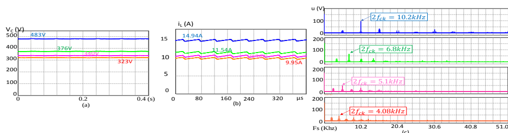
Hình 5. Kết quả mô phỏng với V_S=55V , u_{rms}=110V các kỹ thuật nhiều sóng mang, nét vẽ xanh dương, xanh lá, tím và đỏ là tương ứng với kỹ thuật 2, 3, 4 và 5 sóng mang; (a) điện áp trên tụ DC link, (b) dòng điện ngõ ra i_L và (c) phổ tần điện áp pha tải
