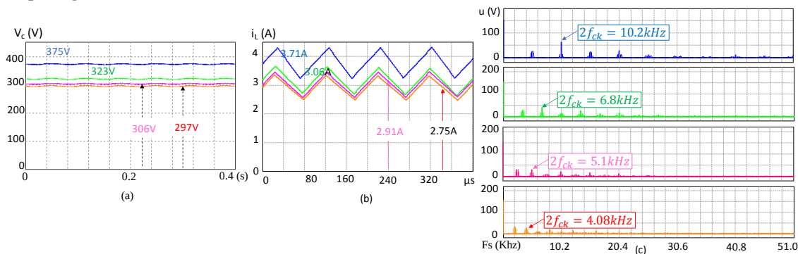
Hình 7. Kết quả mô phỏng với V_s=165V , u_{rms}=110V các kỹ thuật nhiều sóng mang, nét vẽ xanh dương, xanh lá, tím và đỏ là tương ứng với kỹ thuật 2, 3, 4 và 5 sóng mang; (a) điện áp trên tụ DC link, (b) dòng điện ngõ vào i_L và (c) phổ tần điện áp pha tải
