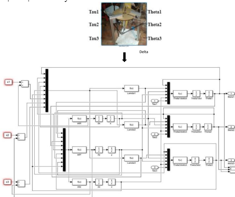
Hình 2. Mô hình động lực học chuyển động của robot Delta 3 - DOF xây dựng trong MATLAB/Simulink và kết cấu cơ khí mô hình robot thực mà tác giả chế tạo phiên bản 2
