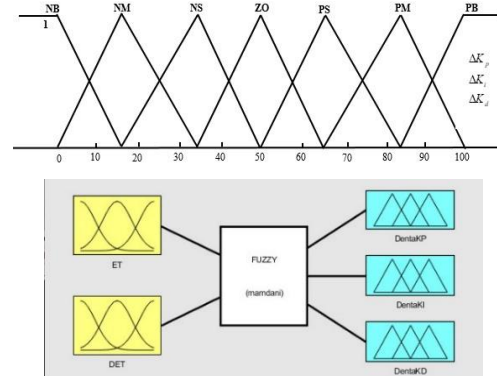
Hình 7. Ngõ ra các hệ số \Delta K_p, \Delta K_i, \Delta K_d và cấu trúc bộ điều khiển mờ
