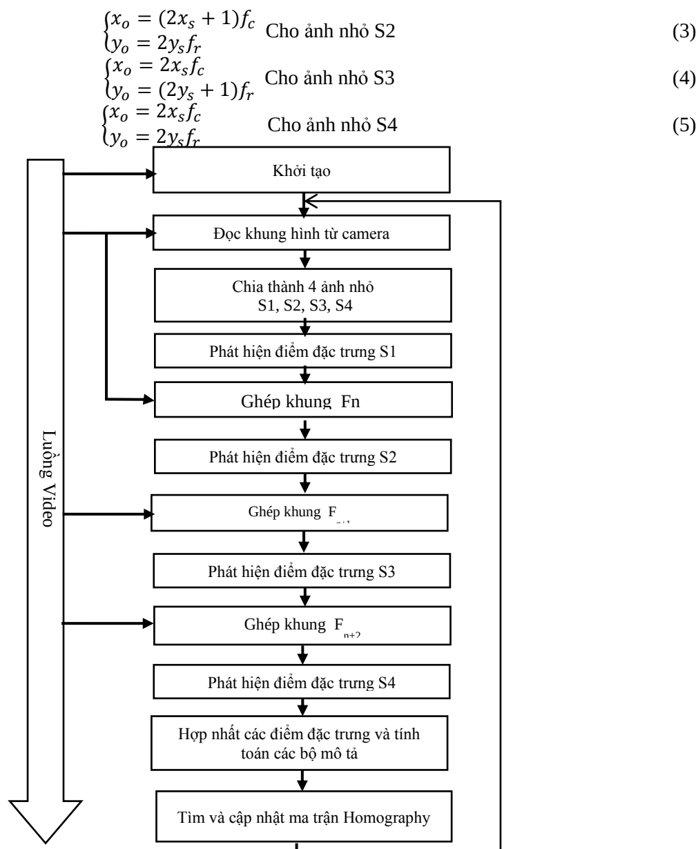
Hình 1. Lưu đồ thuật toán đề xuất tìm ma trận Homography
