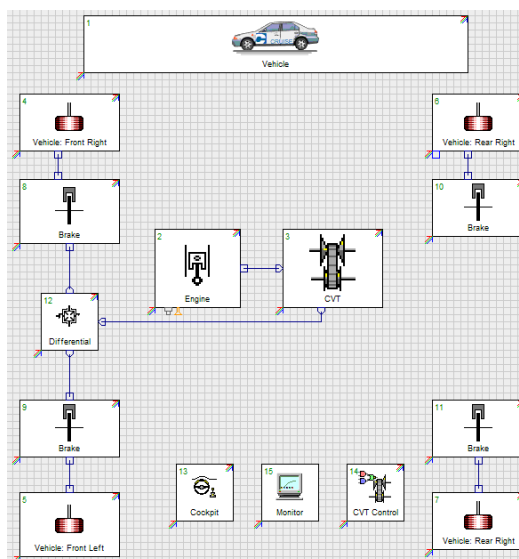
Hình 5. Mô hình mô phỏng xe thông thường trên phần mềm AVL-Cruise
