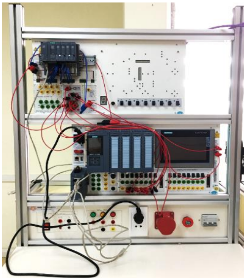
Hình 1. Mô hình thực hành
