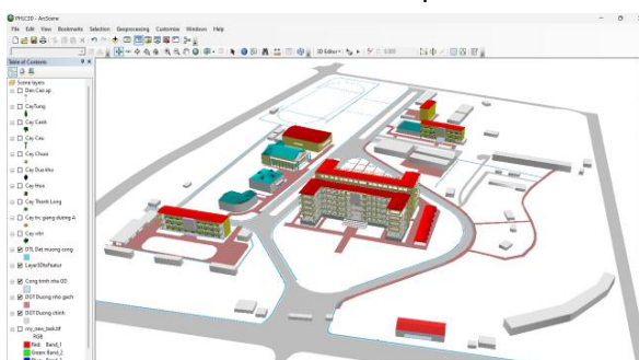
Hình 14. Mô hình 3D một số công trình xây dựng của Phân hiệu trên ArcScene
