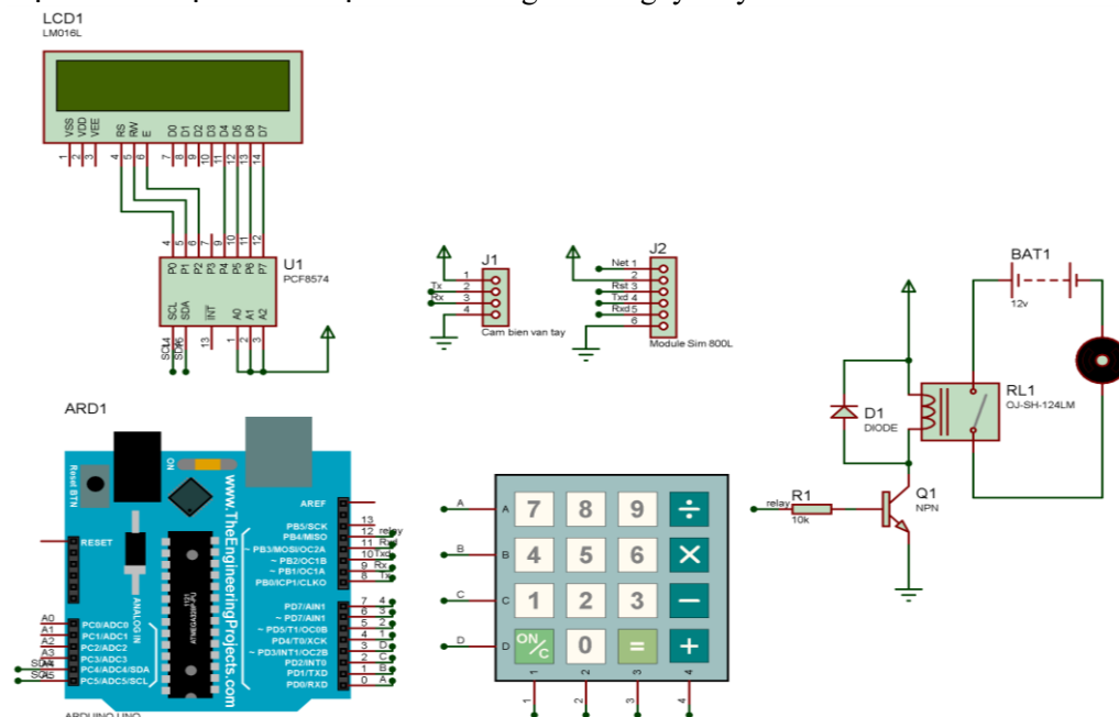
Hình 3. Sơ đồ mạch nguyên lý mạch mô phỏng khóa bảo mật đa lớp trên Proteus
