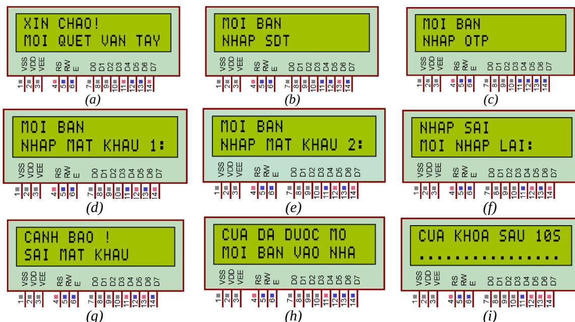
Hình 4. Hoạt động của hệ thống: (a) Yêu cầu quét vân tay; (b) Yêu cầu nhập số điện thoại đã đăng ký; (c) Yêu cầu điện mã OTP gửi về số điện thoại; (d) Yêu cầu nhập mật khẩu lớp 1; (e) Yêu cầu nhập mật khẩu lớp 2; (f) Cảnh báo nhập sai; (g) Cảnh báo truy cập trái phép; (h) Thông tin về cửa được mở khoá thành công; (i) Thông báo cửa sẽ được khoá lại sau 10 giây
