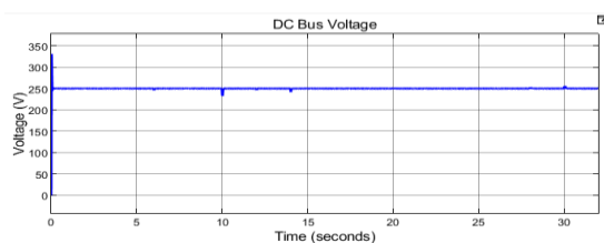
Hình 20. Điện áp DC-bus
