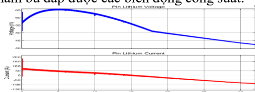
Hình 18. Dòng điện và điện áp của Pin Lithium
