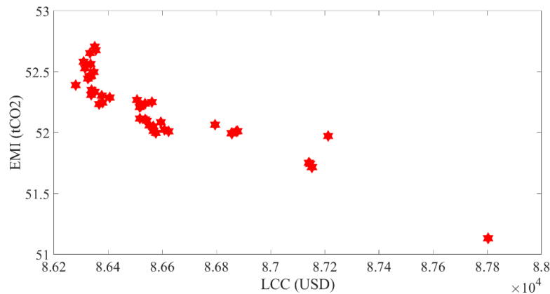
Hình 4. Biểu đồ Pareto chế độ vận hành độc lập ở kịch bản S1
