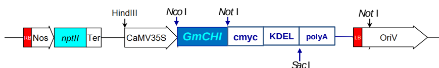
Hình 1. Sơ đồ cấu trúc 35S- GmCHI-cmyc trong vector chuyển gen pCB301. GmCHI trong vi khuẩn A. tumefaciens . nptII : gen kháng kanamycin; CaMV35S : promoter 35S; GmCHI : gene mã hóa chalcone isomerase phân lập từ cây đậu tương; cmyc : trình tự nucleotide mã hóa peptide cmyc; KDEL : trình tự nucleotide mã hóa peptide KDEL
