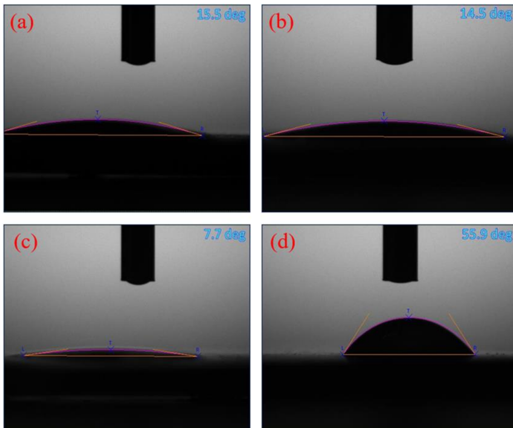
Hình 3. Góc thấm ướt của (a) \text{SrTiO}_3:\text{Er}^{3+}/0,5\%\text{Yb}^{3+} , (b) \text{SrTiO}_3:\text{Er}^{3+}/1\%\text{Yb}^{3+} , (c) \text{SrTiO}_3:\text{Er}^{3+}/2\%\text{Yb}^{3+} , và (d) Ti
