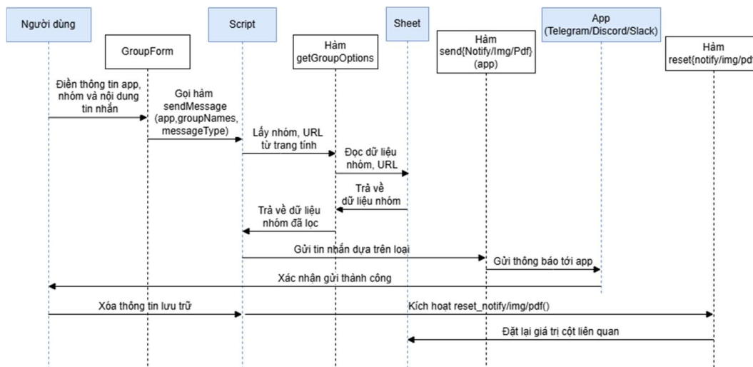
Hình 2. Quy trình quản lý gửi tin nhắn và cập nhật trạng thái hệ thống
