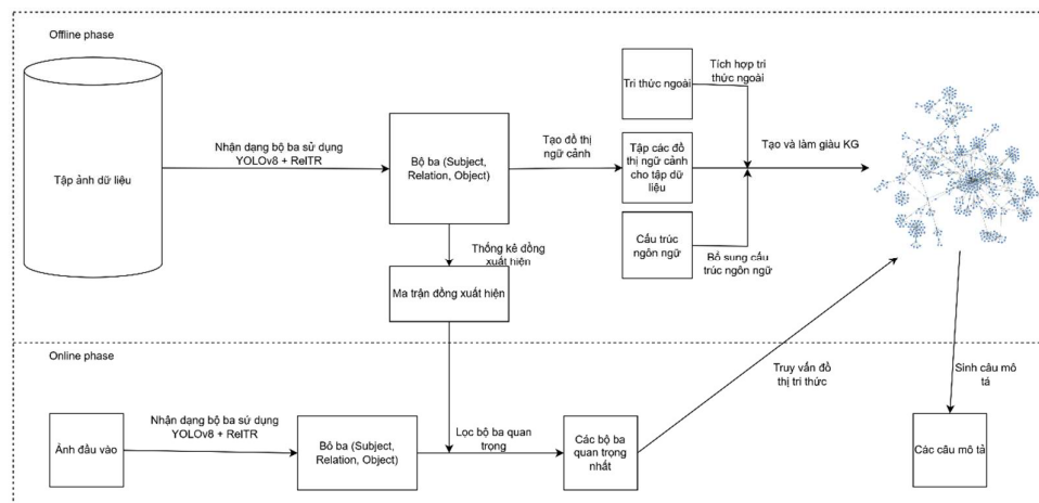
Hình 1. Mô hình mô tả ảnh sử dụng đồ thị tri thức và mạng học sâu
