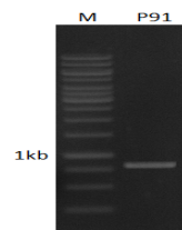
Hình 2. Ảnh điện di sản phẩm PCR nhân đoạn gen matK của mẫu KSTN27 trên gel agarose 1%, M: marker 1kb
