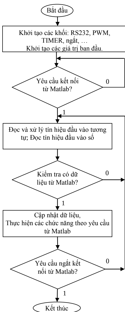
Hình 5. Lưu đồ thuật toán chương trình chính
