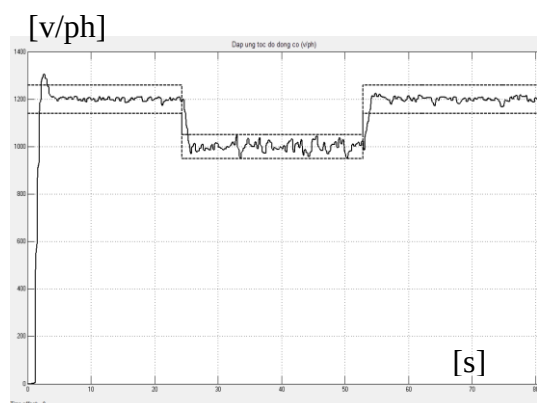
Hình 8. Đáp ứng tốc độ động cơ
