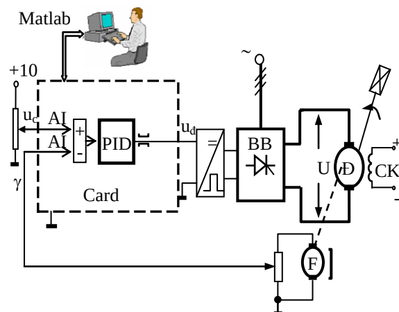
Hình 7. Cấu trúc điều khiển
