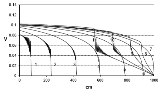
Hình 6. Các đường cong liên tục từ 1 - 11 là các profil biểu diễn vận tốc trong hỗn hợp của freon 21 chứa bọt hơi tương ứng với các khoảng thời gian: t = 5; 15; 28.4; 41.2; 55.4; 66.2; 73.5; 77.3; 82.9; 85 và 85.48 ms
