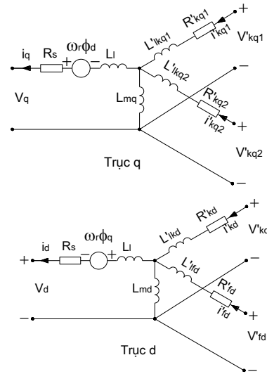
Hình 5. Sơ đồ mạch điện thay thế
