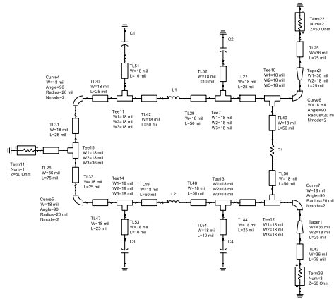
Hình 7. Sơ đồ tương đương mạch dài [6]
