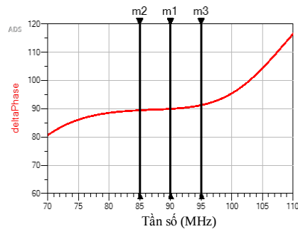
9d) Sai lệch pha giữa hai cổng P2, P3
