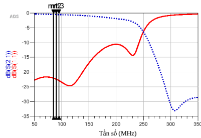
6b) Kết quả mô phỏng bộ lọc LPF
