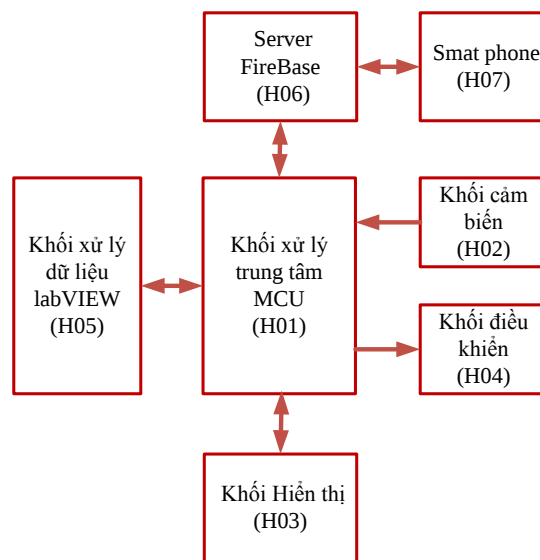
Hình 1. Sơ đồ khối hệ thống
