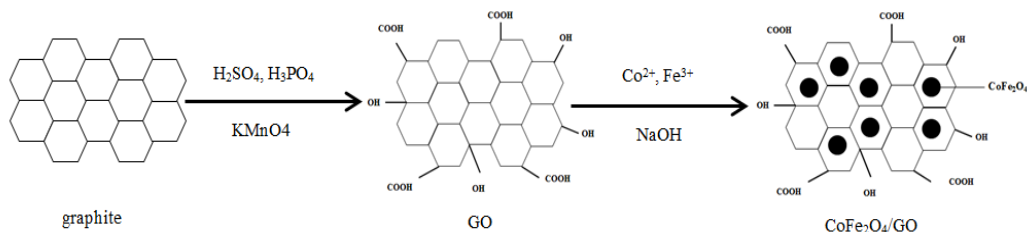
Hình 1. Sơ đồ mô tả quá trình tổng hợp vật liệu nano tổ hợp \text{CoFe}_2\text{O}_4/\text{GO}
