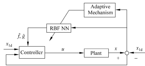
Hình 1. Sơ đồ cấu trúc điều khiển
