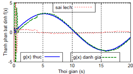
Hình 3. Đánh giá thành phần bất định f(x)
