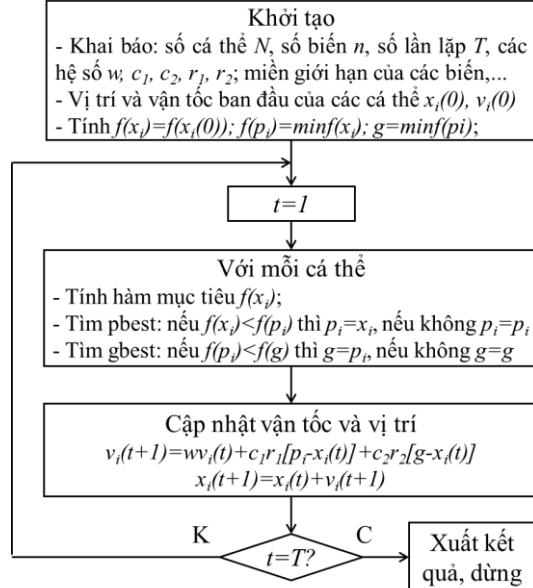
Hình 5. Sơ đồ thuật toán tổng quát của PSO MÔ HÌNH TỐI ƯU HOÁ CHẾ ĐỘ CẮT
