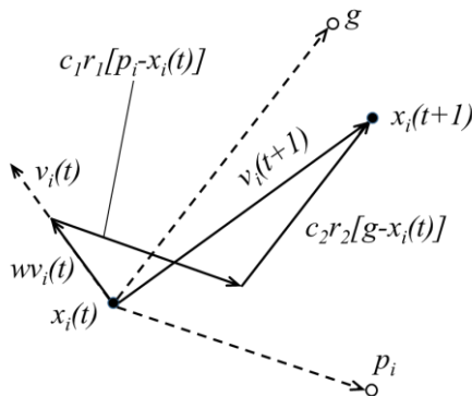
Hình 4. Mô tả giải thuật cập nhật vận tốc và vị trí Vị trí tốt nhất của con thứ i ứng với giá trị nhỏ nhất của hàm mục tiêu (bài toán cực tiểu) mà nó đạt được:
