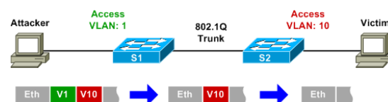
Hình 8. VLAN Hopping with Double Tagging
