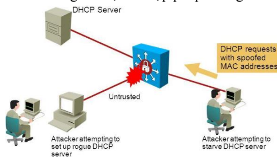
Hình 4. Tấn công kiểu DHCP spoofing
