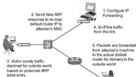
Hình 3. Tấn công kiểu ARP spoofing
