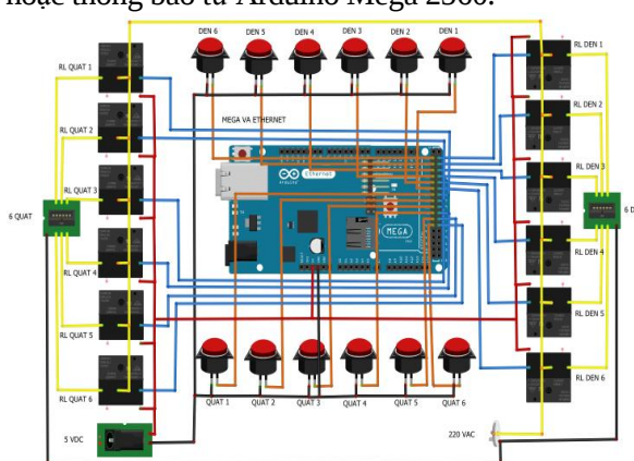
Hình 2. Sơ đồ mạch điện của hệ thống
