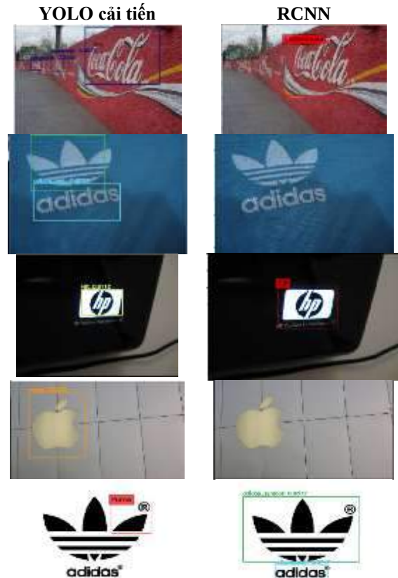
Hình 8. Kết quả dò tìm chính xác bởi YOLOv3 cho những logo biến dạng
