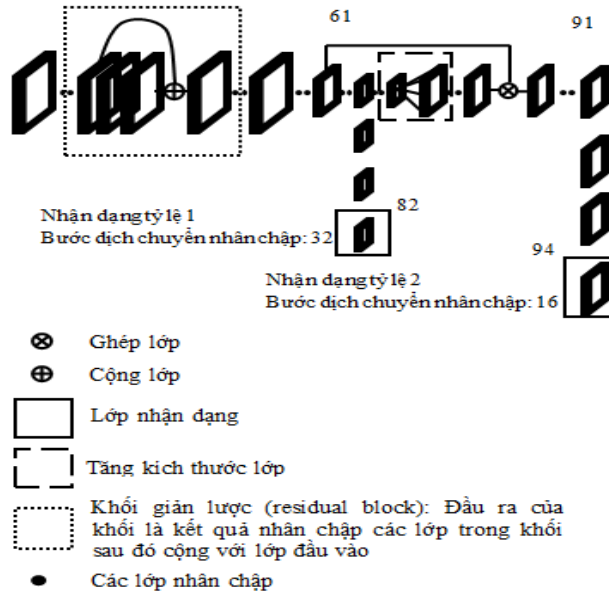
Hình 5. Kiến trúc mạng
