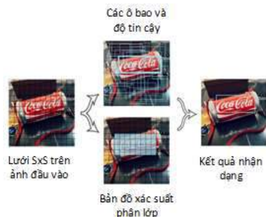
Hình 3. Quy trình thuật toán YOLO
