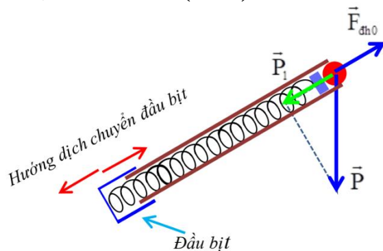
Hình 4. Cơ cấu hiệu chỉnh \Delta l_0
