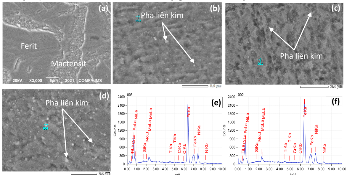
Hình 2. Ảnh tổ chức tế vi của các mẫu thép: (a) mẫu ban đầu; (b) mẫu sau tôi và hóa già trong 2 giờ; (c) mẫu sau tôi và hóa già trong 4 giờ; (d) mẫu sau tôi và hóa già trong 6 giờ; (e) và (f) lần lượt theo thứ tự là phổ EDX của các điểm kiểm tra 003 và 004
