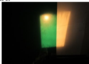
Hình 2. Chiếu ánh sáng vàng và xanh lục vào bì xanh lục
